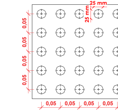
DET. PISO TÁTIL DE ALERTA
