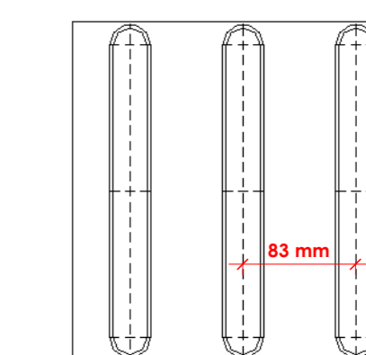
DET. PISO TÁTIL DIRECIONAL
