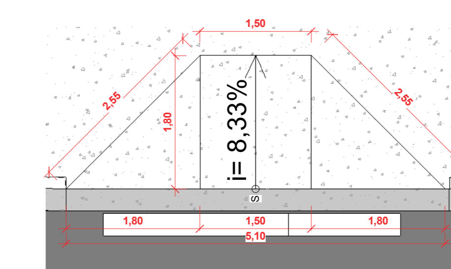
3 Det. Rampa para pedestre 1 : 50
