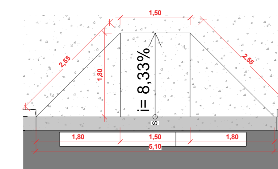
3 Det. Rampa para pedestre 1:50
