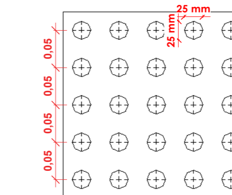
DET. PISO TÁTIL DE ALERTA
